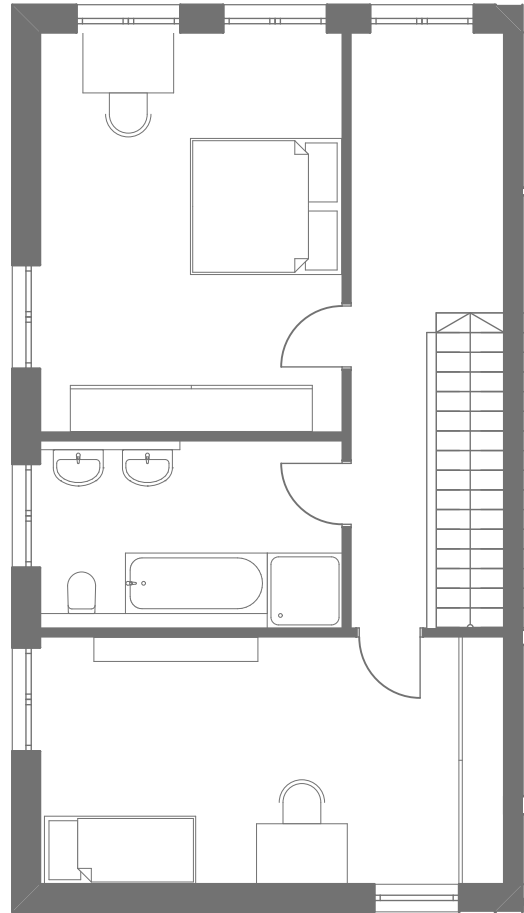
WE 1 - Obergeschoß
